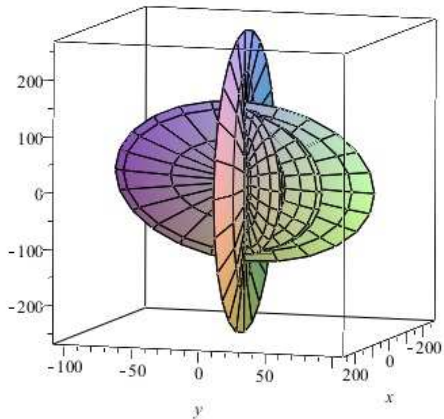
The exact soltuion
