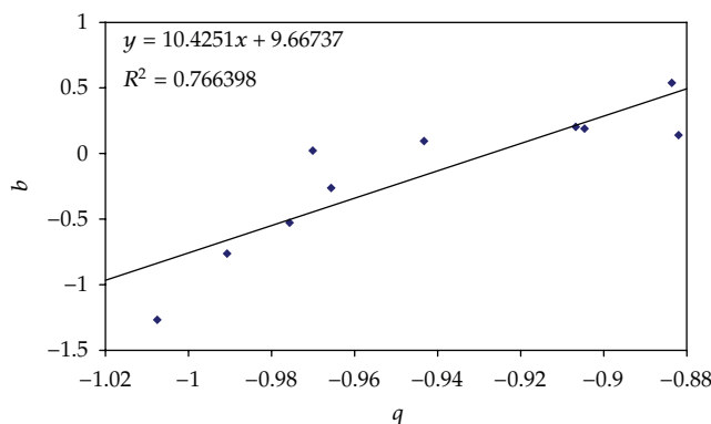
Figure 8: Parameter b values versus parameter q values, for all indices.
